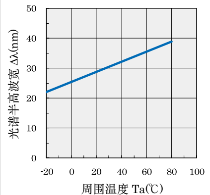
图 9. 光谱半高波宽温度特性
