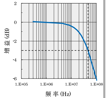
图 6. 频率响应特性
