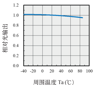
图 5. 相对光输出温度特性
