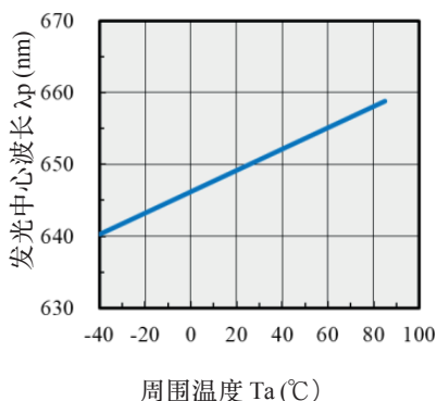
图 8. 发光峰值波长温度特性
