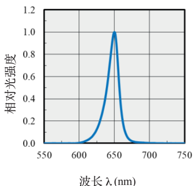
图 7. 发光光谱
