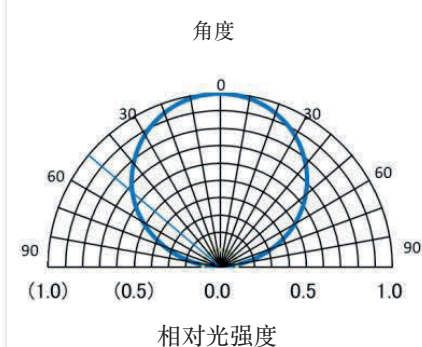
图 6. 指向特性
