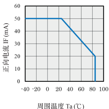
图 1. 降额曲线
