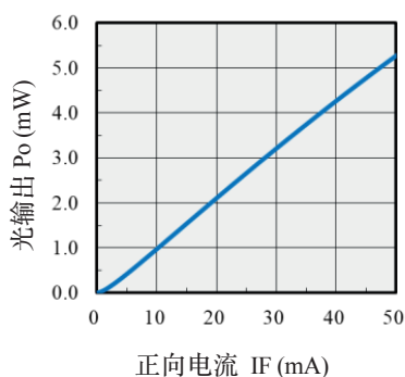
图 4. 正向电流光输出特性
