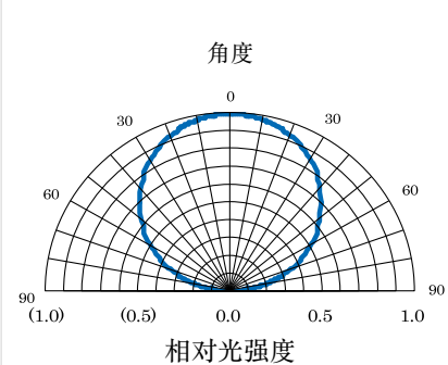
图 6. 指向特性
