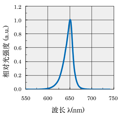
图 7. 发光光谱
