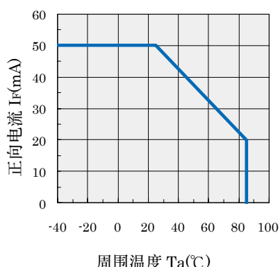
图 1. 降额曲线
