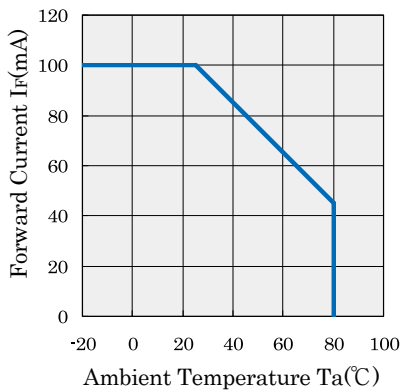
Fig1. I_F / T_a
